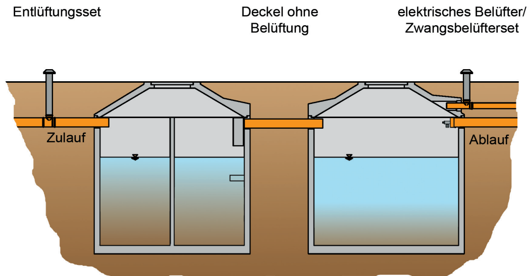
Abb. 6 Zwangsbelüftung/-entlüftung
