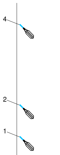
Abb. Zwei-Pumpensteuerung mit zwei Schwimmerschalter
